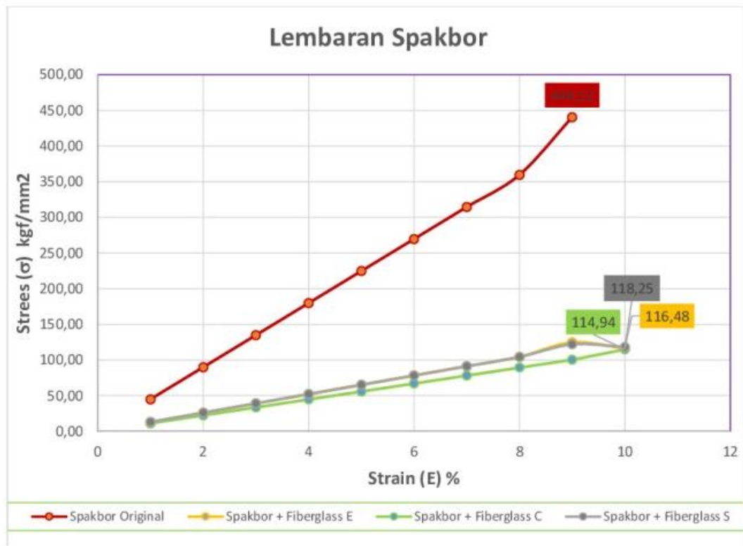
Gambar 3. Grafik Rata-Rata Uji Bending Spakbor Motor
