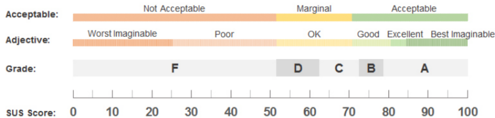
Gambar 17. Penentuan Hasil Penilaian dengan menggunakan Acceptability, Grade Scale, dan Adjective Rating ( https://measuringu.com/interpret-sus-score/ )
