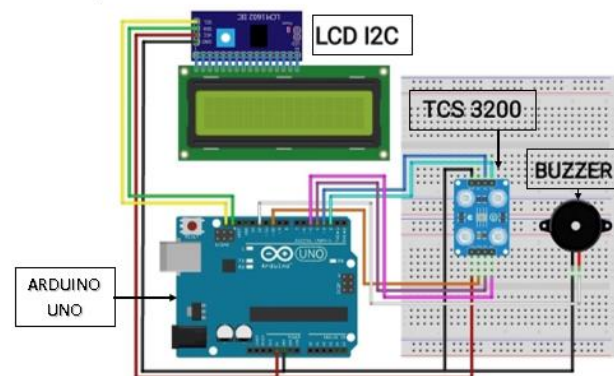
Gambar 4. Skematik Rangkaian
