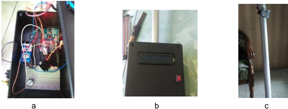
Gambar 5. Tampilan Perangkat Keras
