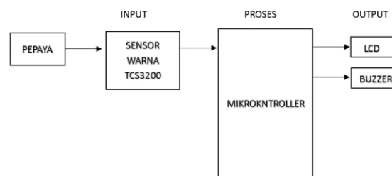
Gambar 1. Diagram Blok Rangkaian
