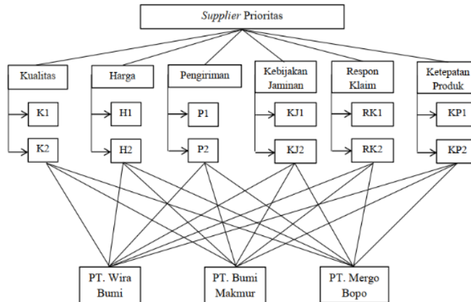
Gambar 2. Struktur Hierarki
