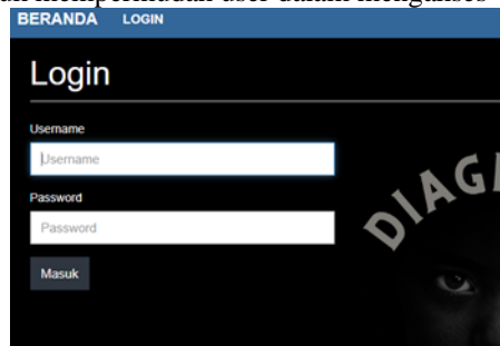
Gambar 6. Menu Login
