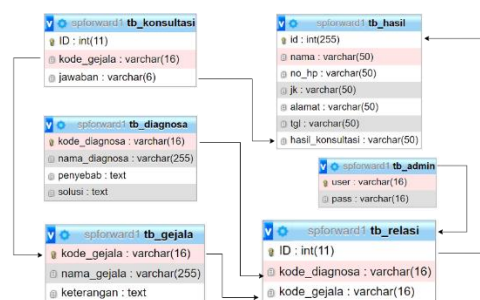
Gambar 5. Relasi Tabel
