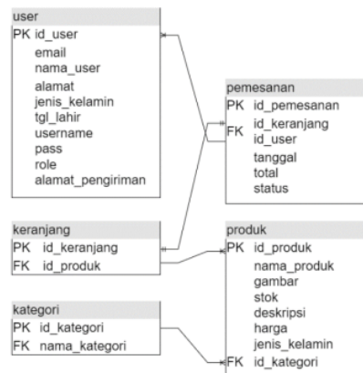
Gambar 4 Relasi Tabel Database
