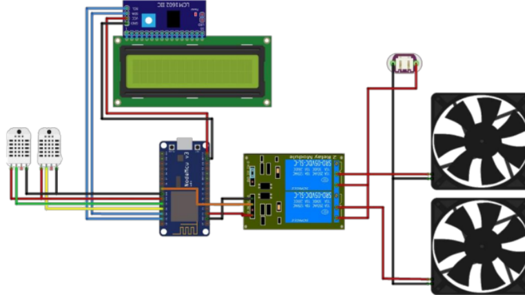
Gambar 6. Rangkaian Wiring Keseluruhan Alat
