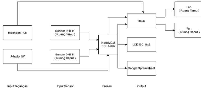
Gambar 2. Blok Diagram Sistem Sekarang
