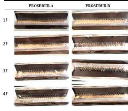
Gambar 3. Hasil Pengelasan
