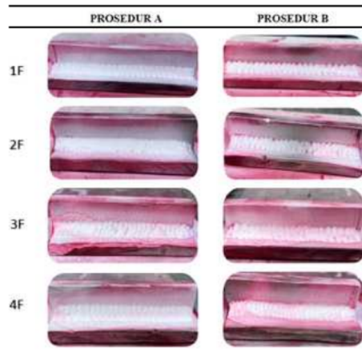
Gambar 2. Hasil Pengelasan dan Pengujian Penetrant Test
