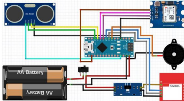
Gambar 11. Rangkaian alat
