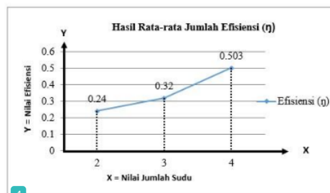
Gambar 8. Grafik Rata-rata Jumlah Sudu Dengan Efisiensi.
