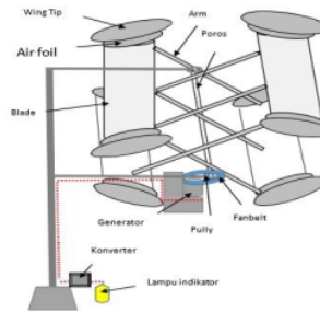
Gambar 3. Desain Alat
