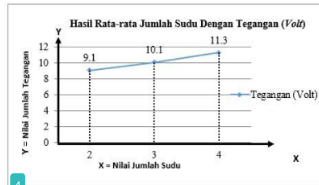
Gambar 6. Grafik Rata-rata Jumlah Sudu Dengan Tegangan (Volt).
