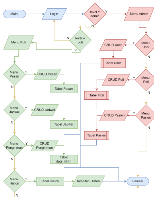
Gambar 3. Flowchart rancang bangun sistem pengingat kontrol dokter dan minum obat
