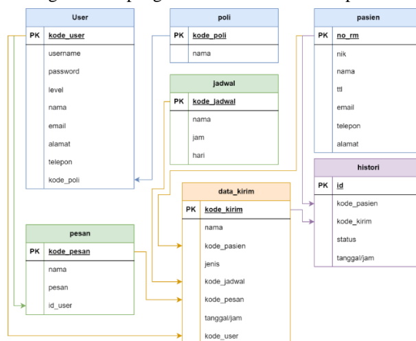
Gambar 4. ERD sistem pengingat kontrol dokter dan minum obat
