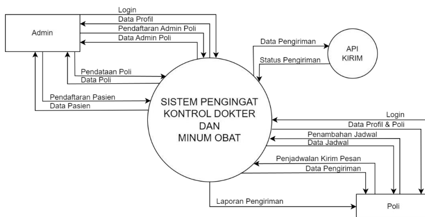
Gambar 5. DFD sistem pengingat kontrol dokter dan minum obat
