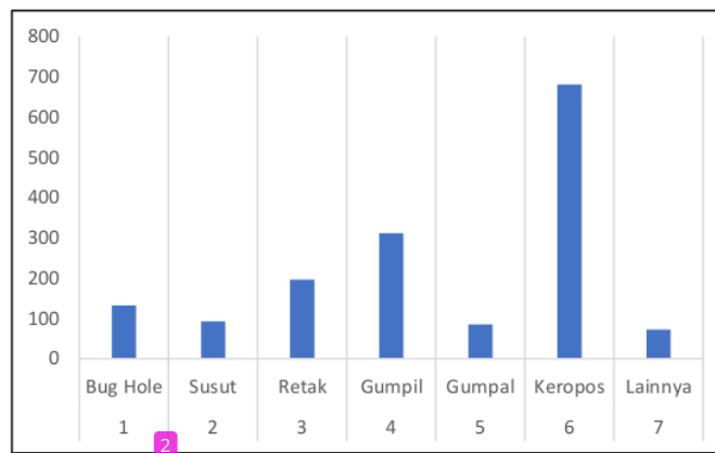
Gambar 3. Histogram Kecacatan Produksi Beton
