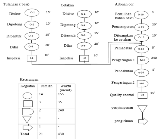
Gambar 2. Peta Aliran Proses
