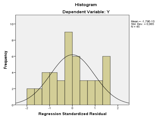
Gambar 1 : Uji Histogram
