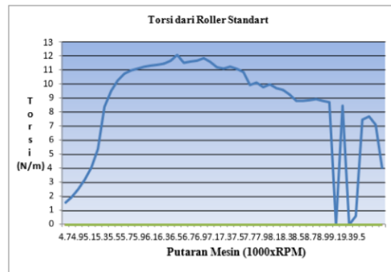
Gambar 4. Torsi dari roller standart
