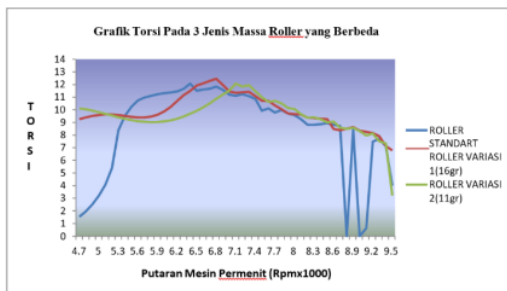
Gambar 9. Torsi pada 3 jenis massa roller yang berbeda
