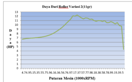
Gambar 6. Daya Dari Roller Variasi 2 (11 gr)
