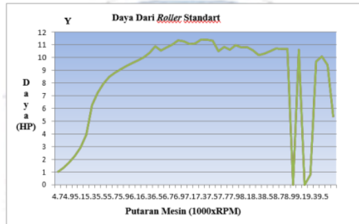
Gambar 3. Daya dari roller standart
