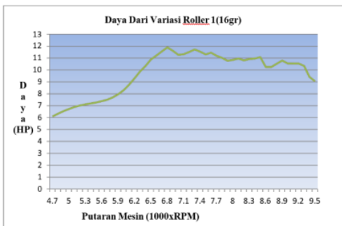
Gambar 4. Daya Dari Roller Variasi 1 (16gr)
