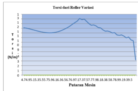
Gambar 7. Torsi Dari Roller Variasi 2 (11gr)
