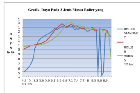
Gambar 8. Daya pada 3 jenis roller yang berbeda
