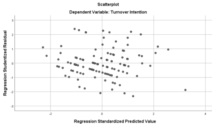
8 Gambar 2. Hasil Uji Heteroskedastisitas
