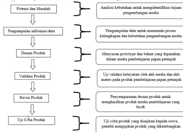
Gambar 1. Model Borg&Gall (1983) [28]
