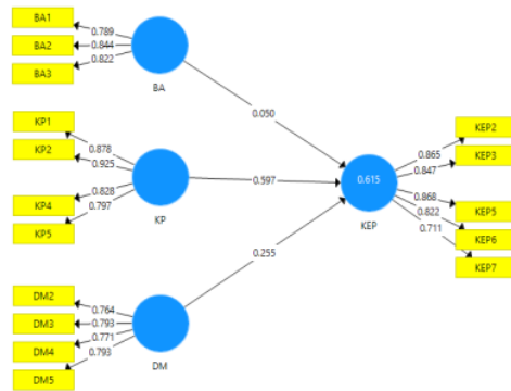
Gambar 5. Model hasil keluaran bootstrapping
