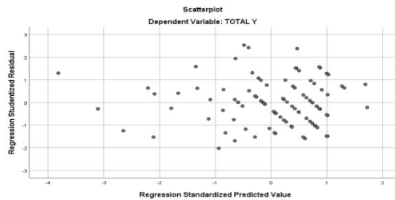
Gambar 2. Hasil Uji Heteroskedastisitas Output Data IBM SPSS 26
