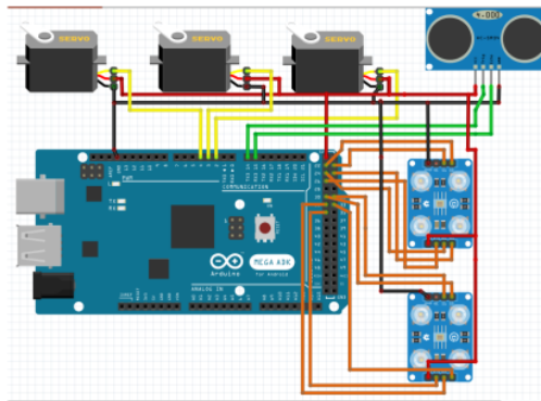
Gambar 1. Pengawatan Keseluruhan Alat
