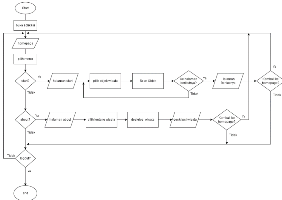
Gambar 3. Flowchart Aplikasi
