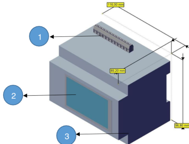
Gambar 4. Desain Alat
