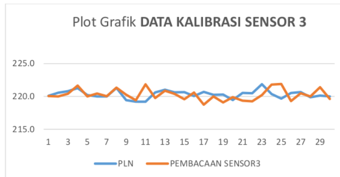
Gambar 17 Hasil pembacaan sensor Phase T
