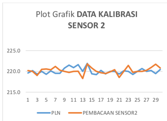
Gambar 14 Hasil pembacaan sensor Phase S
