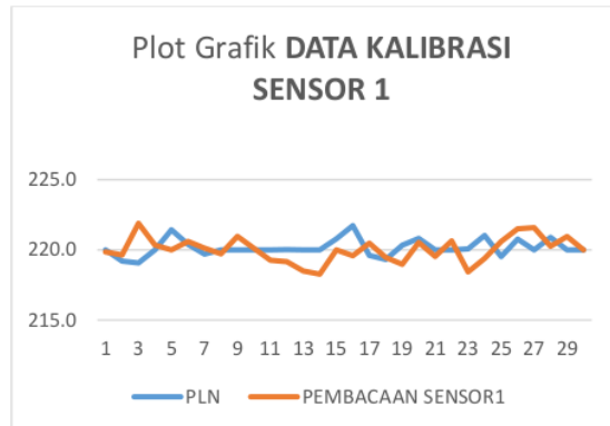
Gambar 11 Pembacaan Sensor Phase R
