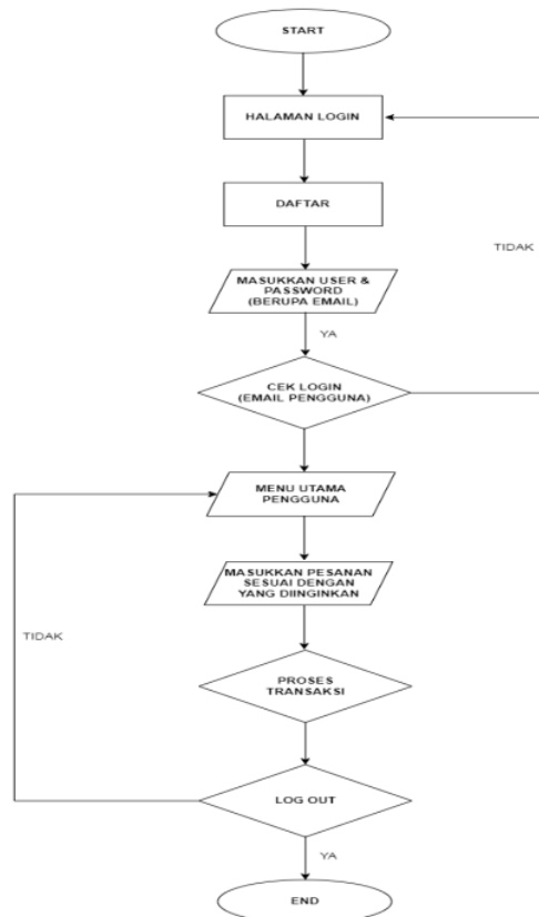
Gambar 2. Flowchart Pengguna
