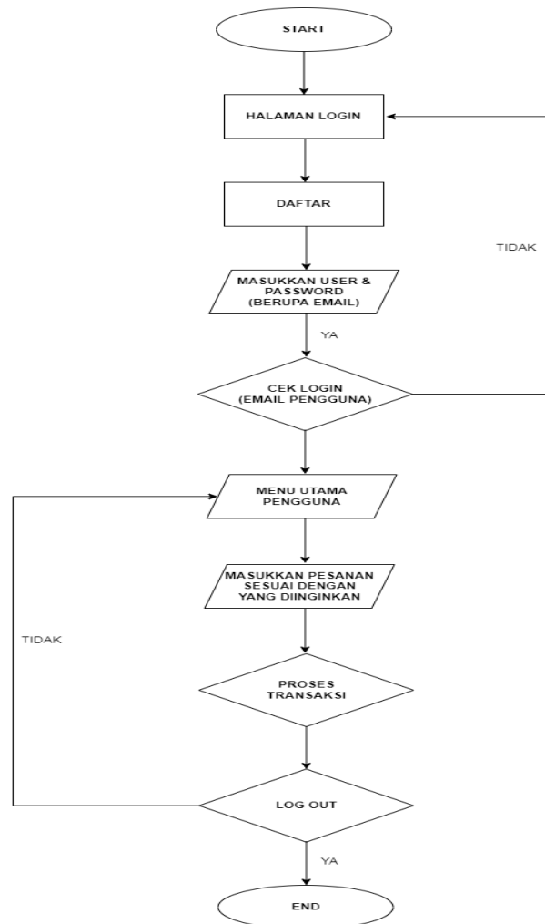
Gambar 2. Flowchart Pengguna
