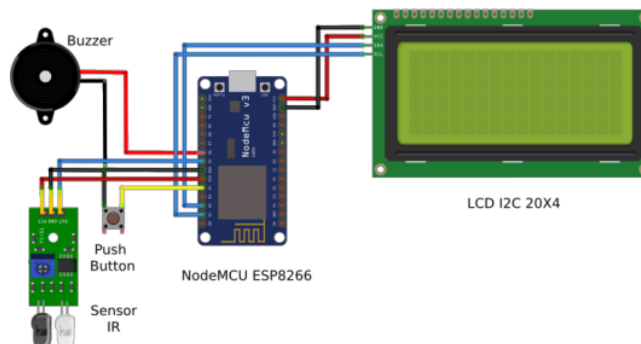
Gambar 3. Wiring Diagram Keseluruhan dari Alat Paper Counter
