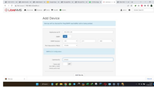
Gambar 6. Halaman Penambahan Perangkat (Add Device)
