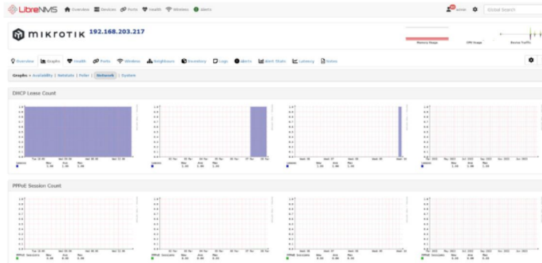
Gambar 13. Grafik network
