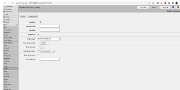
Gambar 3. Konfigurasi SNMP di mikrotik [1]
