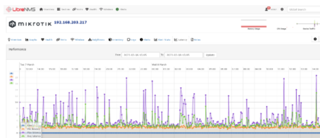
Gambar 9. Grafik latency
