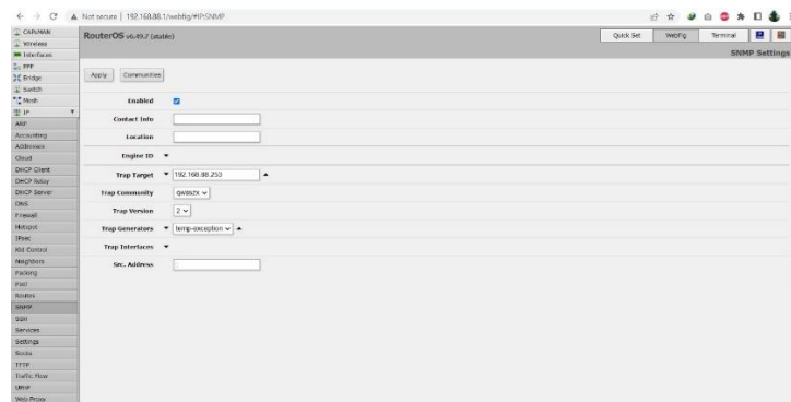
Gambar 3. Konfigurasi SNMP di mikrotik [1]
