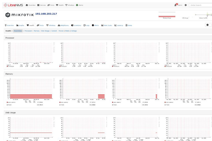
Gambar 11. Grafik resource
