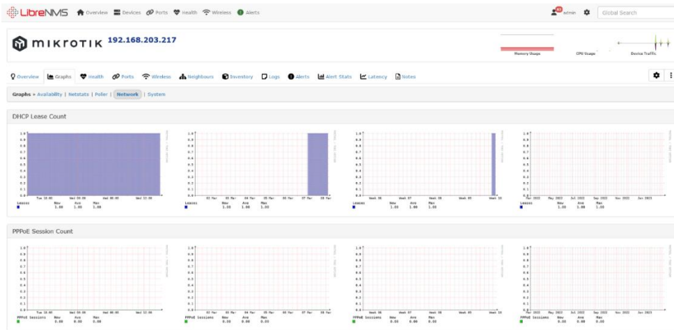
Gambar 13. Grafik network
