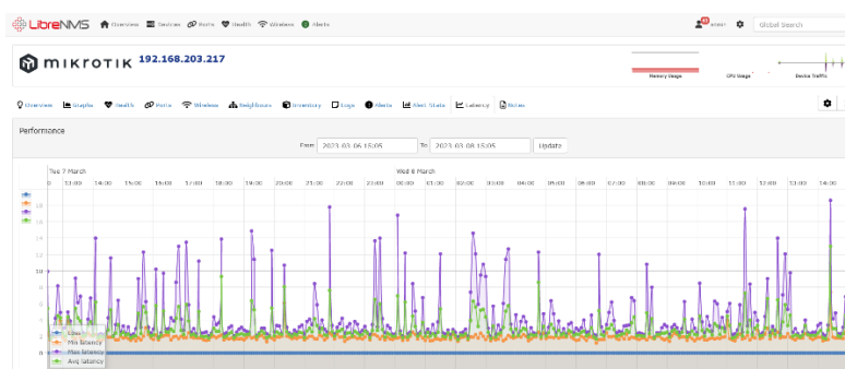
Gambar 9. Grafik latency
