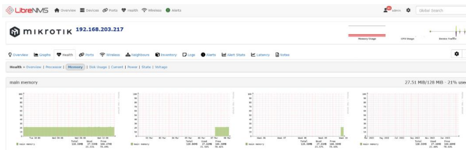
Gambar 12. Grafik memory
