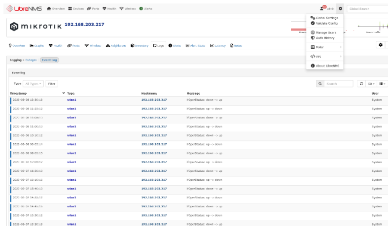
Gambar 10. Log alat
