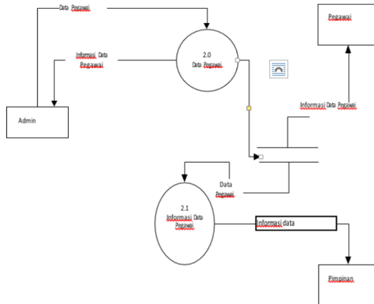
Gambar 5 DFD 1
