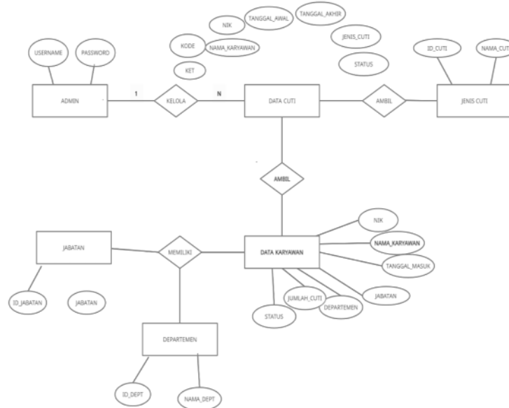
Gambar 6 ERD
