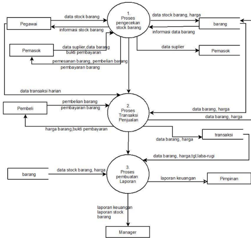
Gambar 1 DFD
