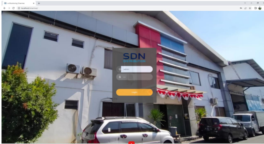
Gambar 8. Halaman Login
