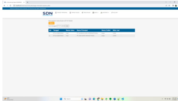
Gambar 16. Halaman Penjualan
