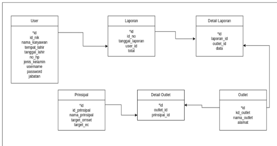
Gambar 7. Tabel Relasi
