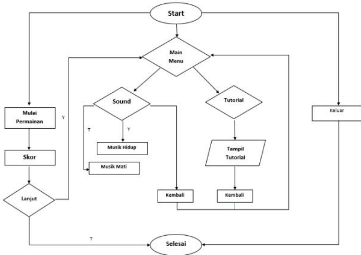
Gambar 1. Flowchart Aplikasi
