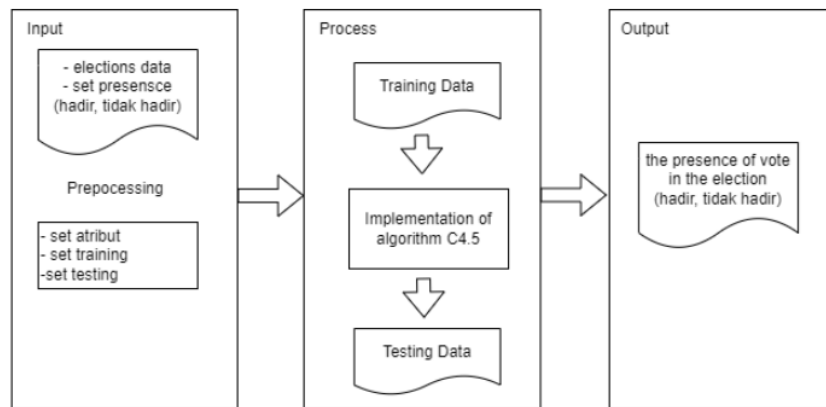
Gambar 1. Diagram Klasifikasi
