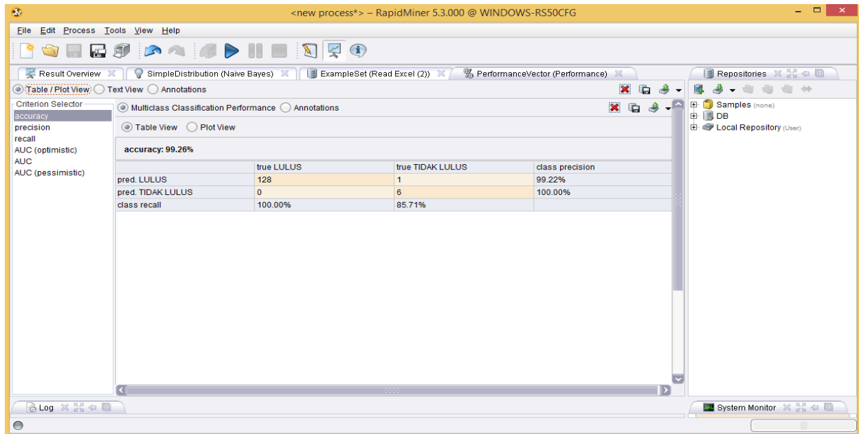
Gambar 12. Nilai akurasi
