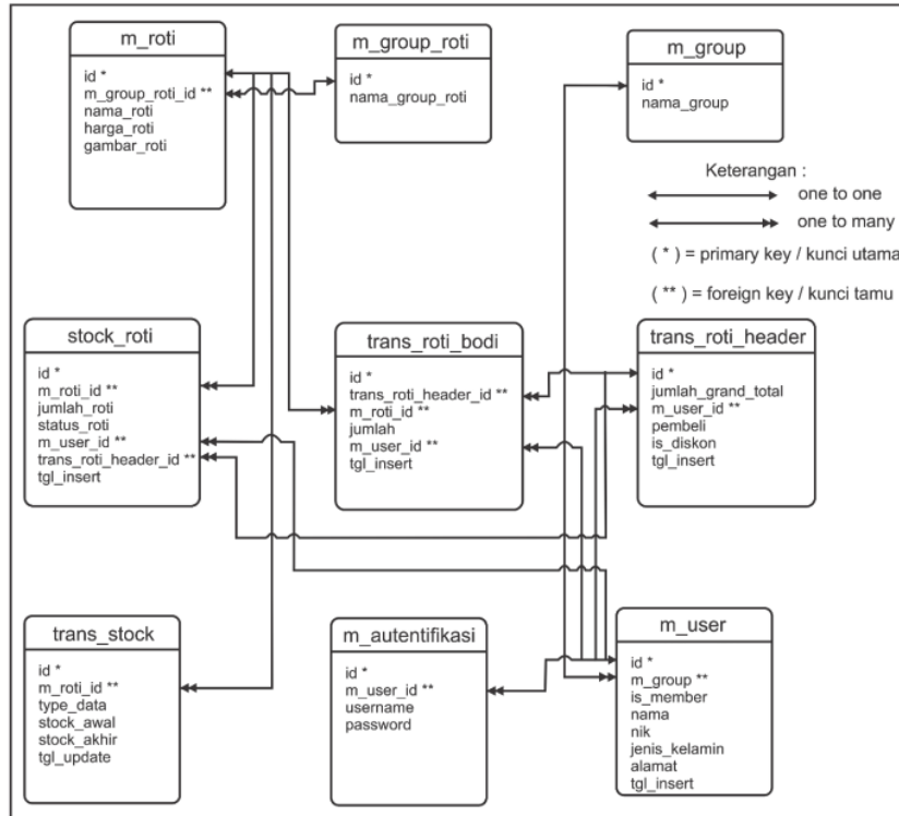
Gambar 6. Tabel Relasi Database
