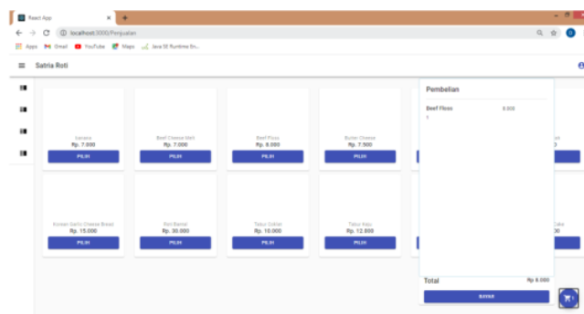
Gambar 11. Pembayaran pesanan
