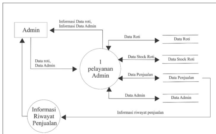
Gambar 5. DFD Sistem
