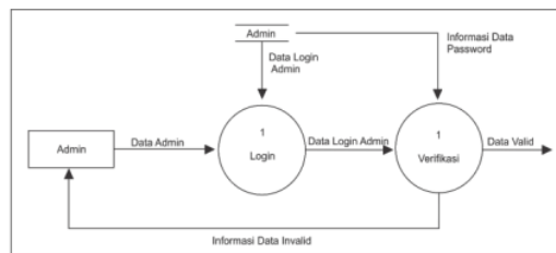
Gambar 4. DFD Login Admin
