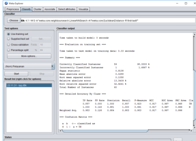
Gambar 8. Hasil Klasifikasi Data Training
