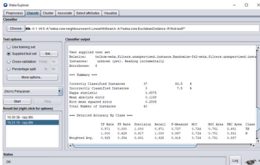
Gambar 14. Hasil Klasifikasi Data Testing
