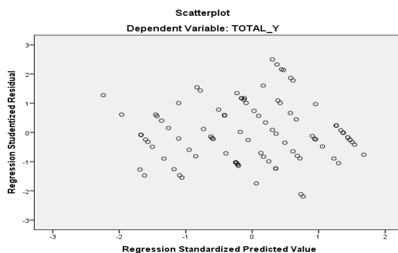
Gambar 2. Hasil Uji Heteroskedastisitas spss 24
