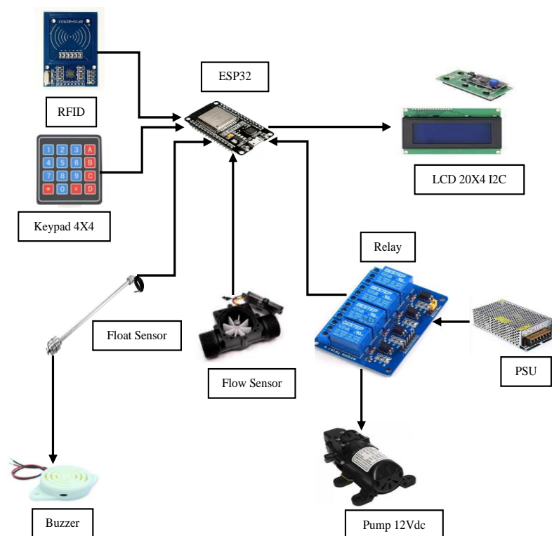
Gambar 3. Ilustrasi desain hardware
