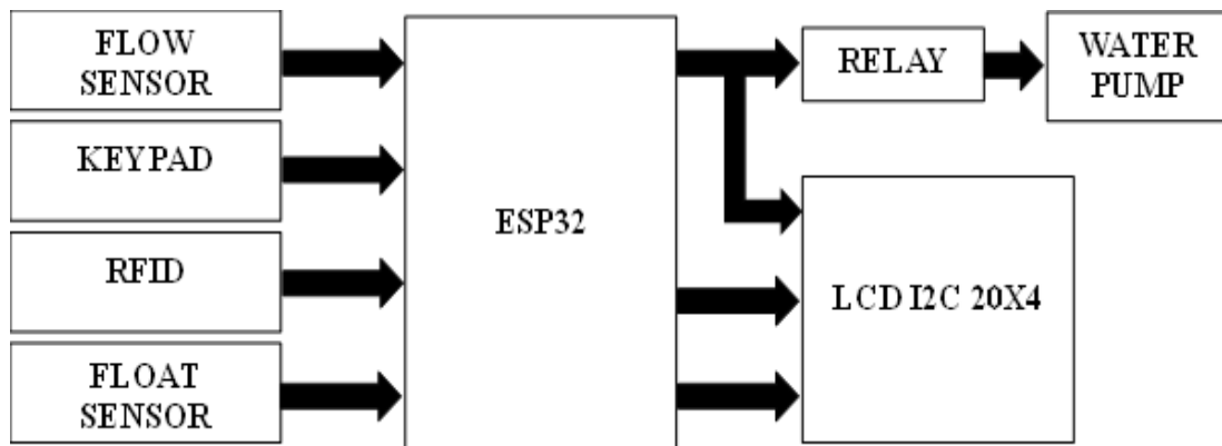
Gambar 2. Ilustrasi desain hardware
