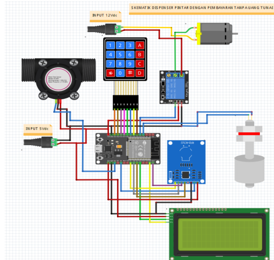
Gambar 5. Skematik Sistem
