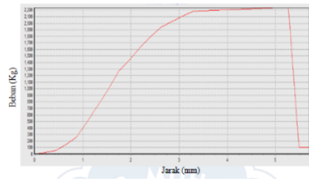
Gambar 7. Grafik Beban Terhadap Jarak Spesimen 2 Suhu Preheating 40°C
