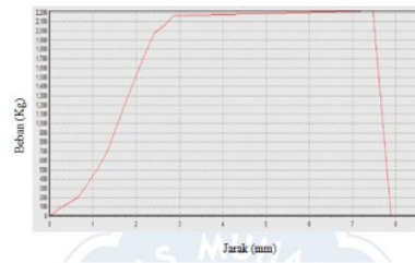
Gambar 4. Grafik Beban Terhadap Jarak Spesimen 1 Tanpa Preheating
