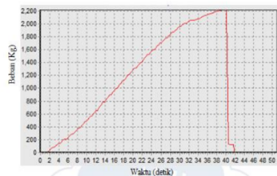
Gambar 2. Grafik Beban Terhadap Waktu Spesimen 1 tanpa Preheating
