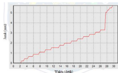
Gambar 6. Grafik Jarak Terhadap Waktu Spesimen 2 Suhu Preheating 40°C
