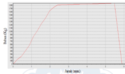
Gambar 10. Grafik Beban Terhadap Jarak Spesimen 3 Suhu Preheating 80°C
