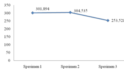
Gambar 11. Grafik Perbandingan Tegangan 3 Spesimen (Spesimen 1= tanpa preheating , Spesimen 2 = suhu preheating 40°C, Spesimen 3 = suhu preheating 80°C)
