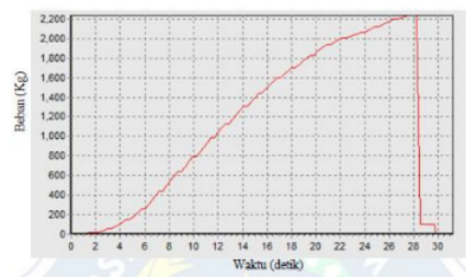
Gambar 5. Beban Terhadap Waktu Spesimen 2 Suhu Preheating 40°C
