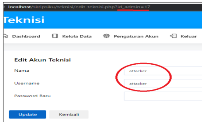
Gambar 10 Halaman Edit Akun
