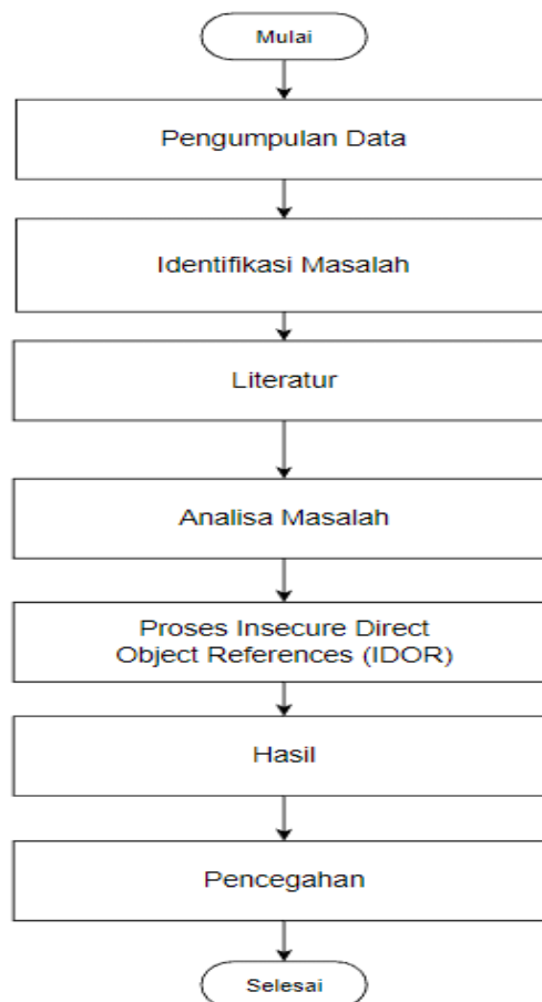
Gambar 1 Teknik Analisa
