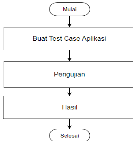
Gambar 2 Perancangan Sistem
