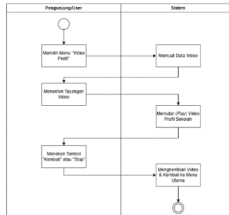
Gambar 6. petunjuk penonton video profil
