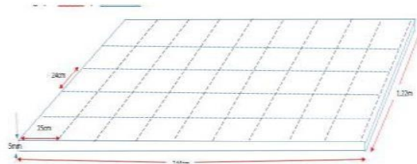
Gambar 2.2 Lembar aluminium 5052 dengan skema pemotongannya
