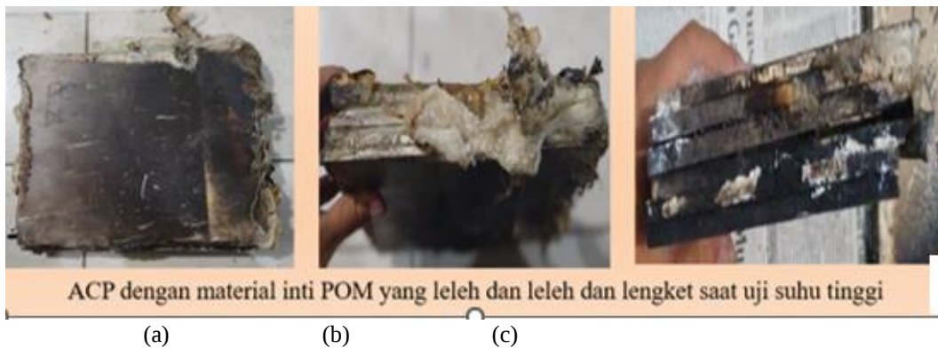
Gambar 3.2 ACP dengan material inti POM setelah uji suhu tinggi, (a) Tampak atas, lengket POM dengan aluminium (b), (c) Tampak samping, meleleh POM menempel ke aluminium
