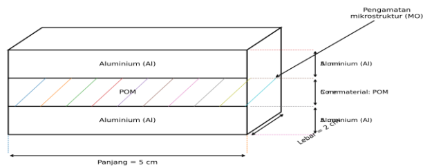
Gambar 2.7 Skema sampel ACP untuk pengamatan mikrostruktur (MO)
