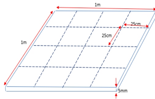
Gambar 2.3 (a) Lembar material Polyoxymethylene (POM) (b) Skema pemotongan lembar POM
