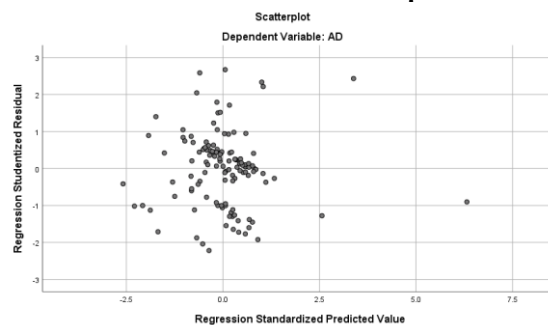
Gambar 2. Grafik Scatterplot
