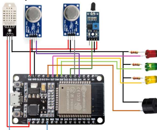
Gambar 5. Skema Rangkaian
