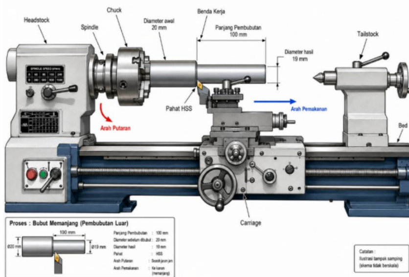
42 Gambar 1. Skema proses pembubutan
