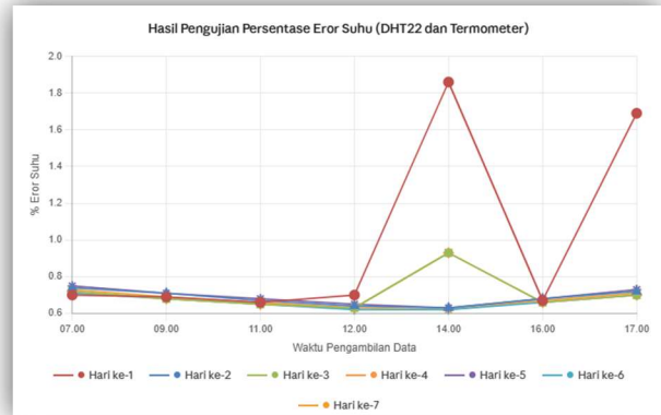
Gambar 7. Grafik % eror suhu kandang
