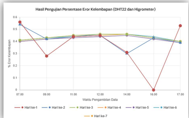
Gambar 9. Grafik % eror kelembapan kandang
