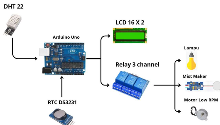
Gambar 2. Perancangan alat
