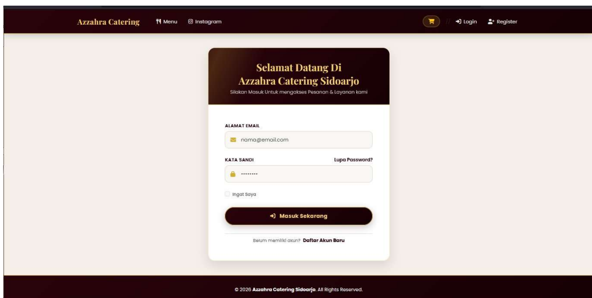
Gambar 3.4 Halaman Login
