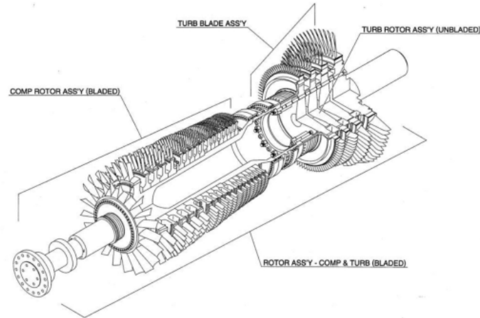
Gambar 4. Komponen pada gas turbin (Sumber: PT. XYZ)
