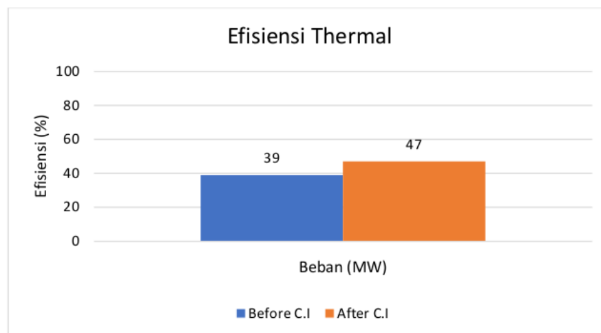
Gambar 8. Efisiensi Thermal
