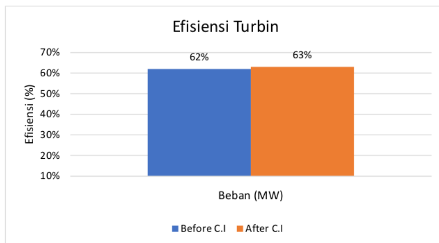
Gambar 10. Efisiensi Turbin
