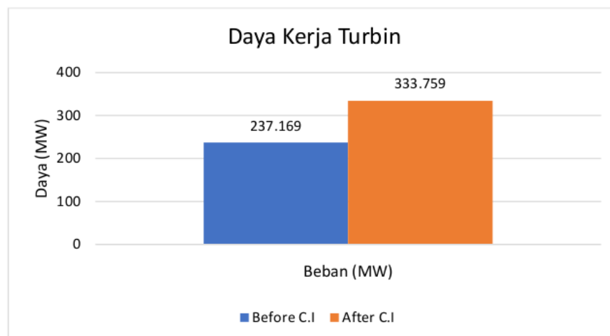
Gambar 6. Daya Kerja Turbin
