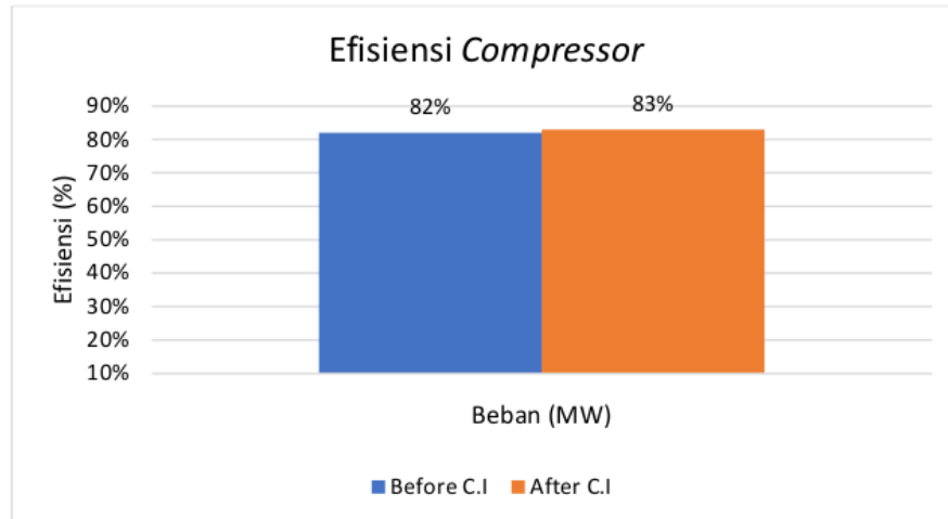
Gambar 9. Efisiensi Compressor
