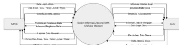
Gambar 5. DFD Level 0 Sistem Informasi Absensi SMK Angkasa Mojosari
