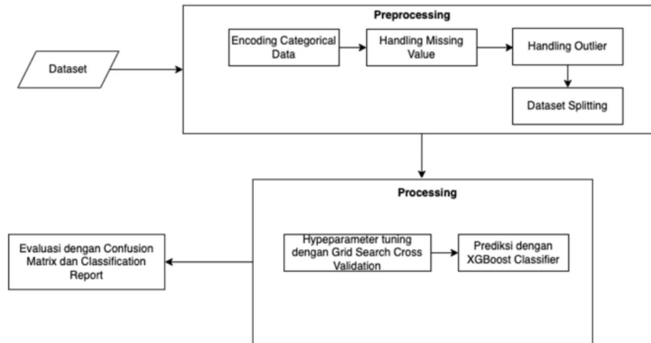
Gambar 1 Tahapan Penelitian
