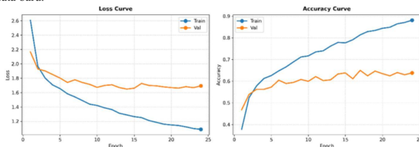
Gambar 5. Plot kurva Loss dan Akurasi pada Epoch 24
