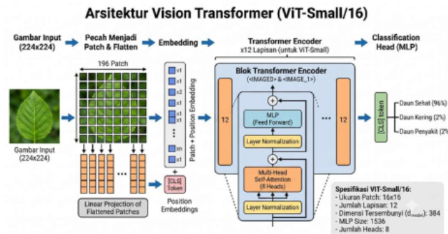
Gambar 2. Arsitektur Vision Transformer
