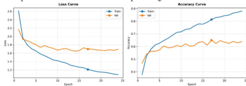
Gambar 4. Plot kurva Loss dan Akurasi pada Epoch 17
