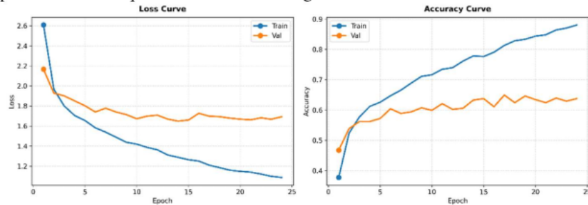
Gambar 3. Plot kurva Loss dan Akurasi pada Epoch 1
